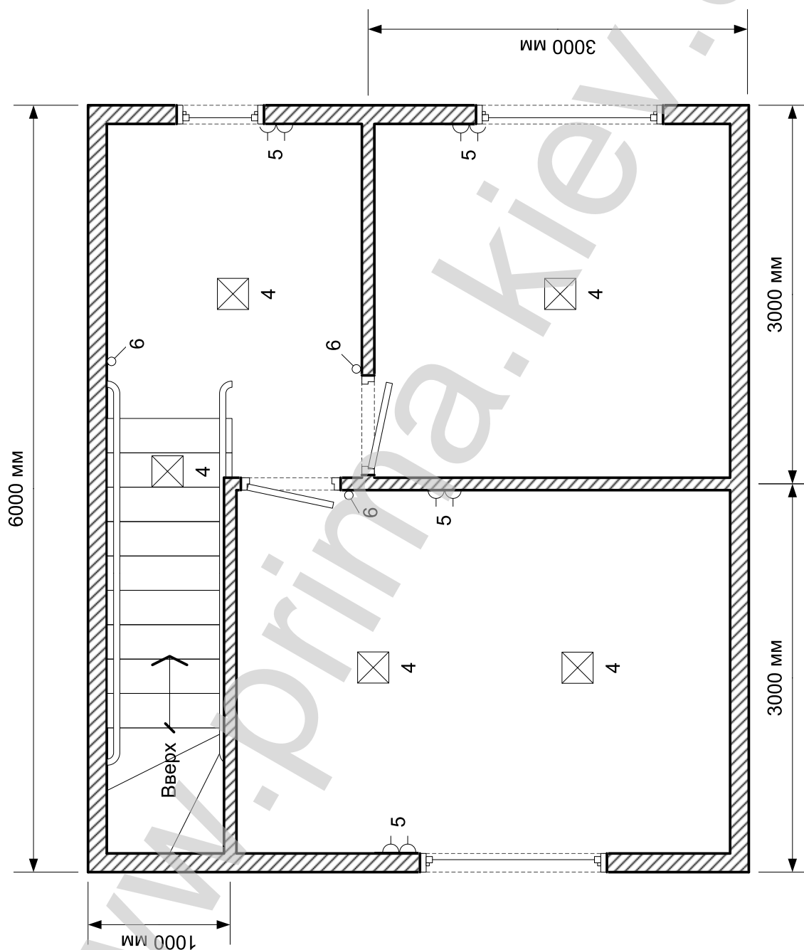
План-схема 2-го этажа изделия:
