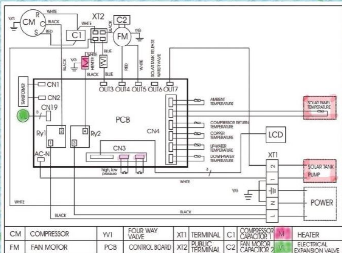
Схема принципиальная электрическая.
