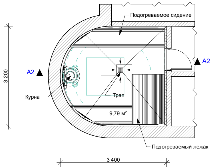
ПЛАН ХАММАМА
