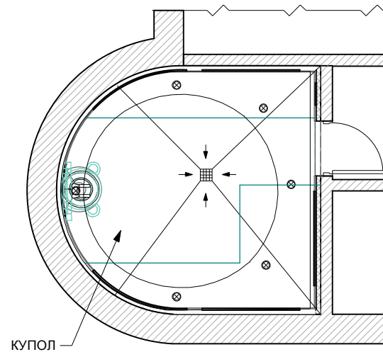
ПЛАН ПОТОЛКА
