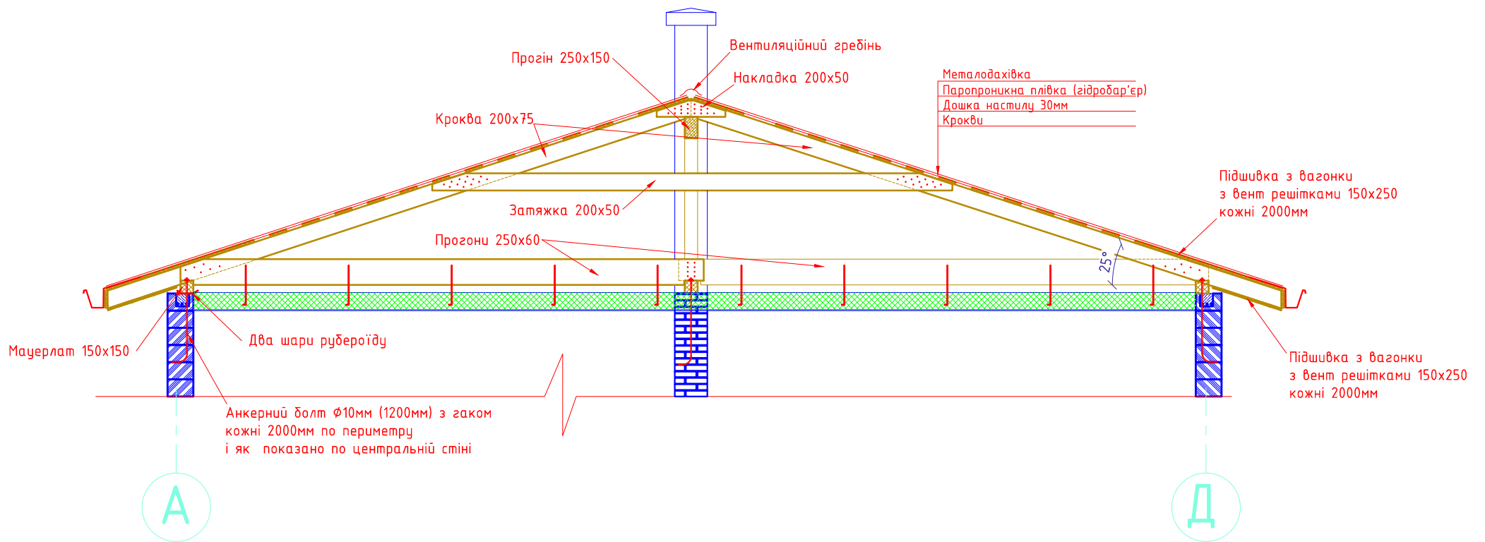
РОЗРІЗ В-В (ПО ДАХУ)
