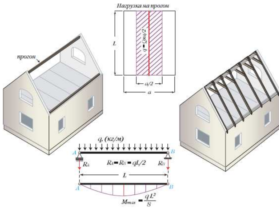
Рис. 24. Пример решения мансардной крыши на коньковых прогонах без дополнительных опор
