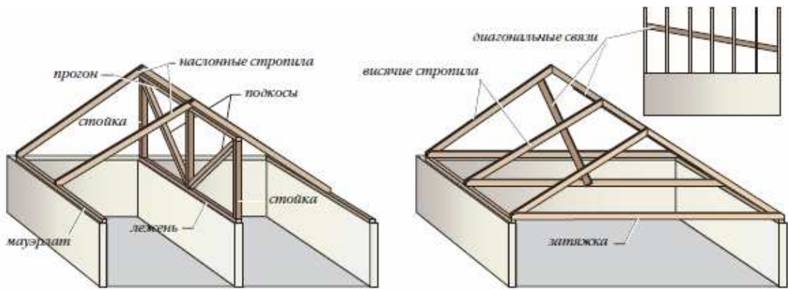
Рис. 12. Пример обеспечения пространственной жесткости
