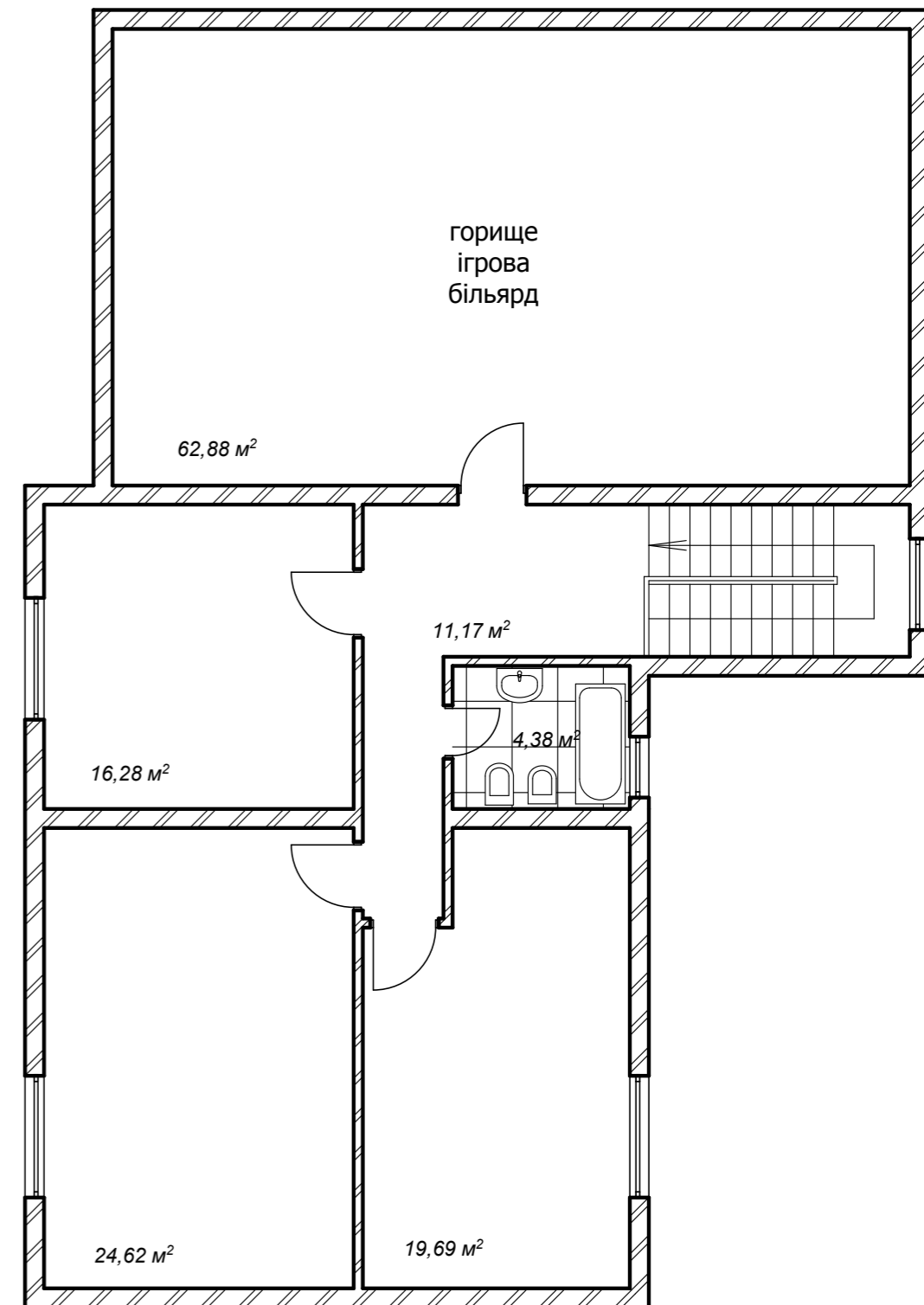
План мансардного поверху
