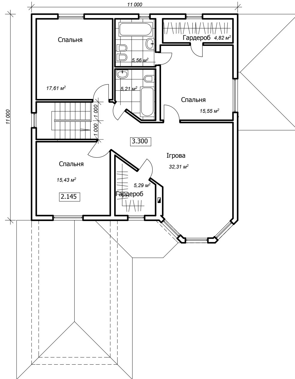
План 2 - го поверху
