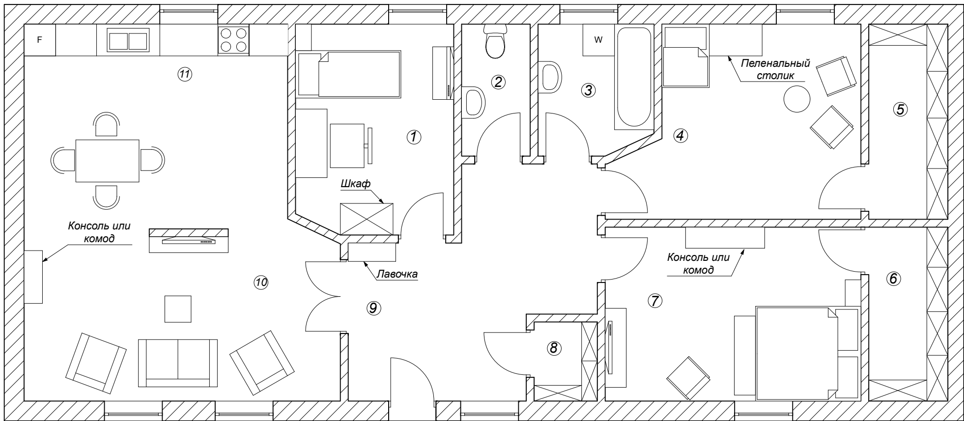
Экспликация помещений
