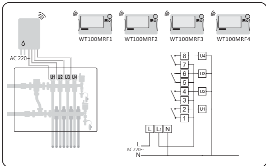
Рис.7: модель WT100MRF
