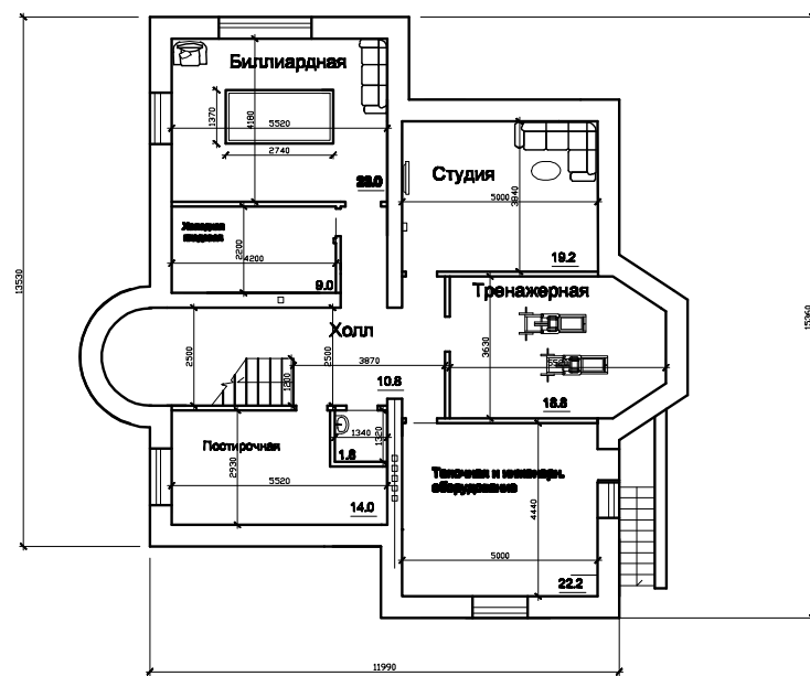
План цокольного этажа на отм. -3.000
