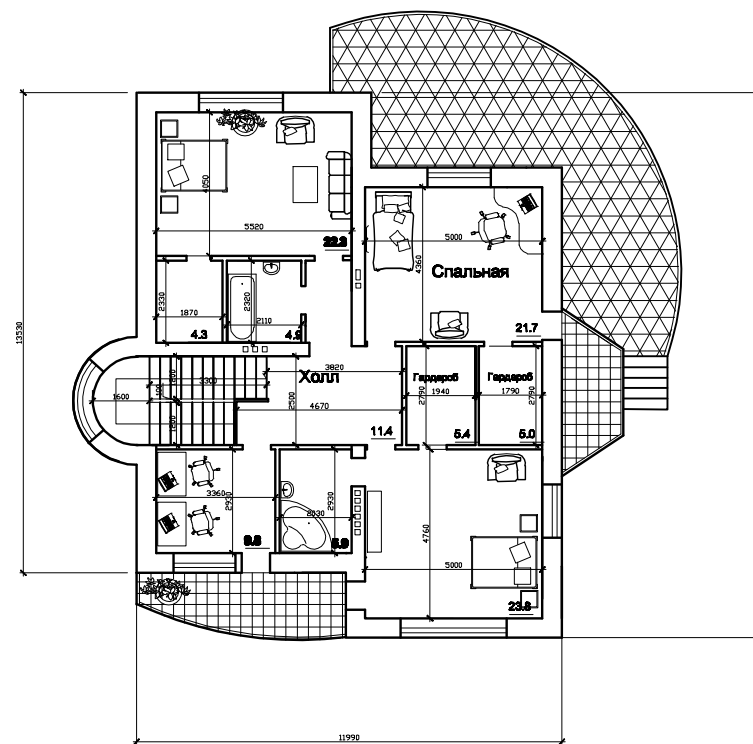
План 2-го этажа на отм. +3.300
