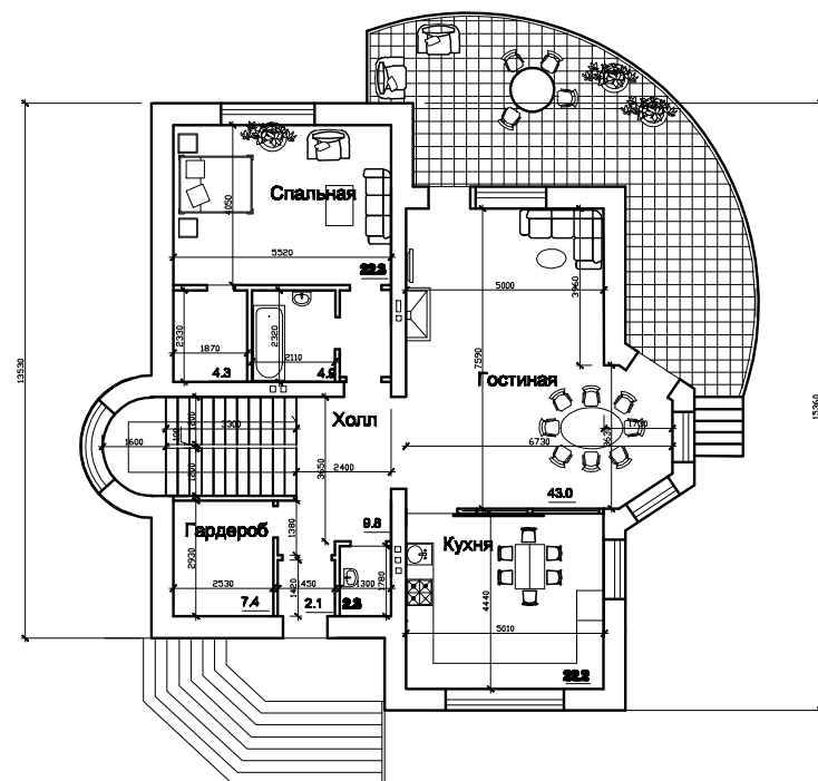
План 1-го этажа на отм. +0.000
