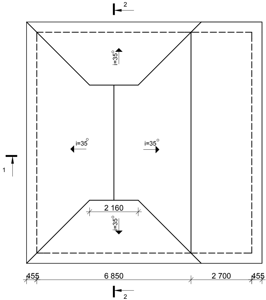
ПЛАН КРОВЛИ М 1:100
