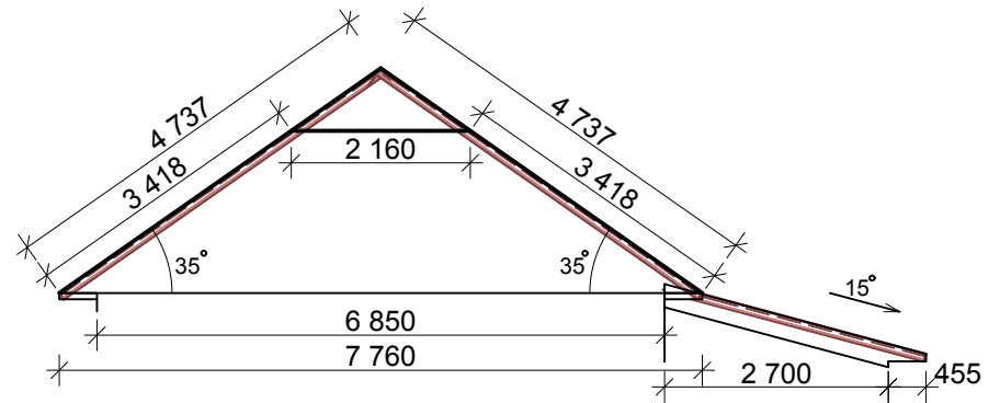
РАЗРЕЗ 1-1 М 1:100
