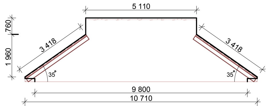
РАЗРЕЗ 2-2 М 1:100
