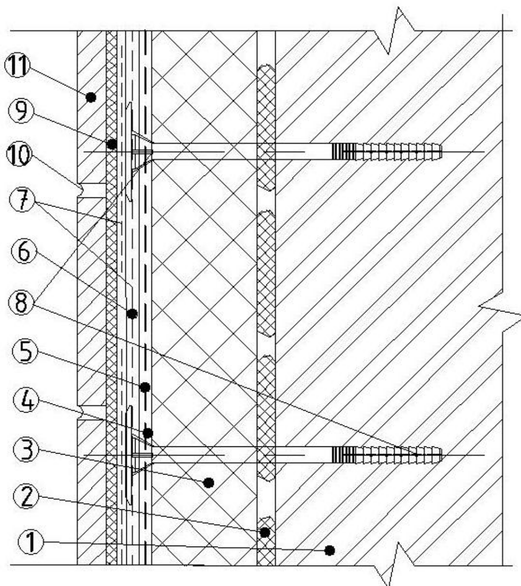
Рисунок 1. Конструктивно-технологическое решение по устройству утепления цоколя системы Baumit:
