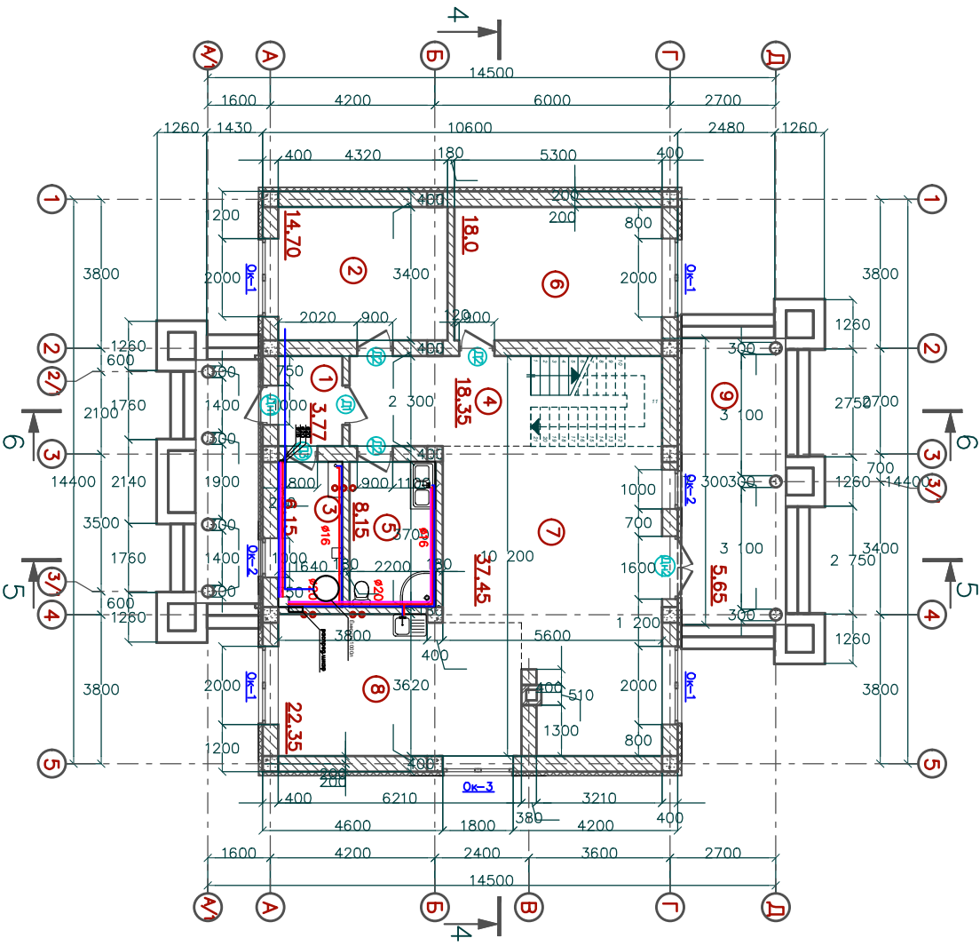
План 1 — 2-го этажа на отм. 0,000
