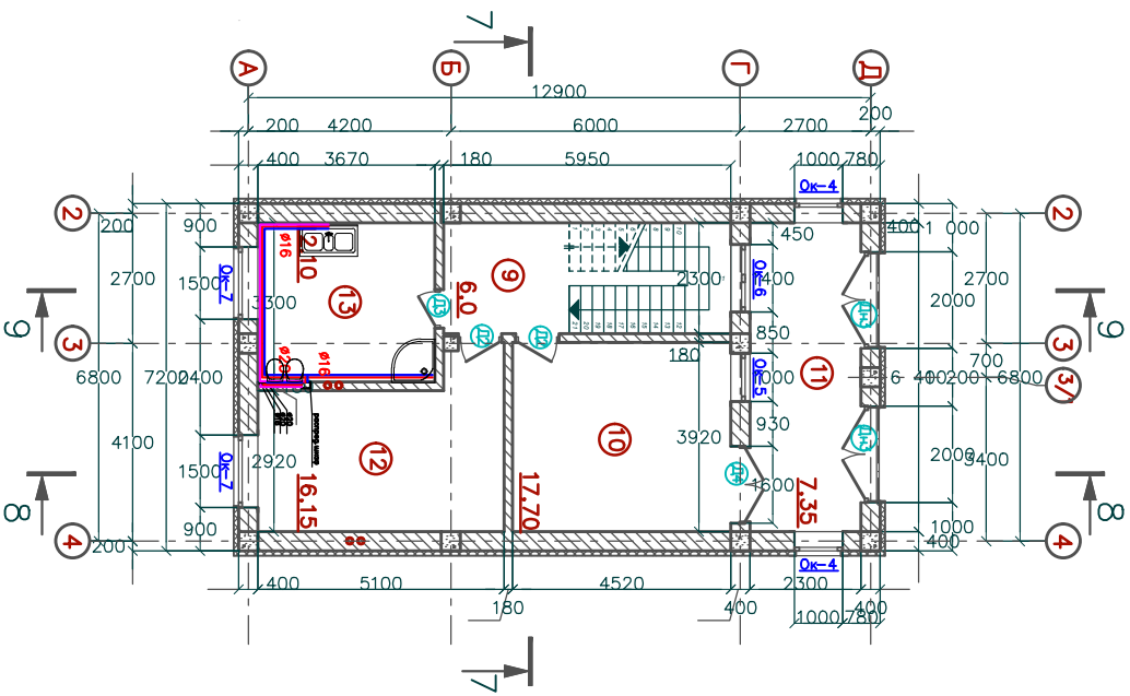
План 2 — 2-го этажа на отм. +3,400
