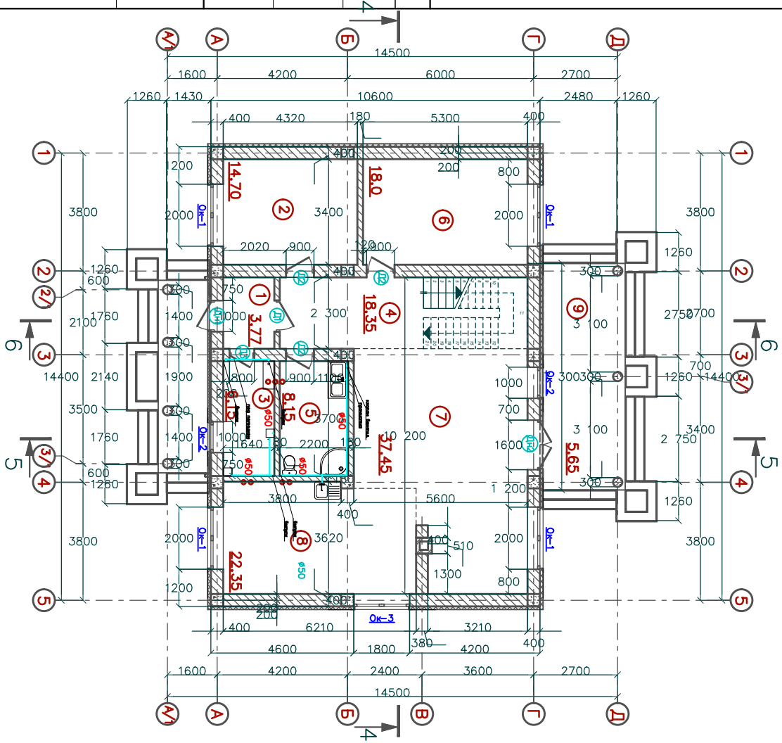
План 1—20 этаж на отм. 0,000
