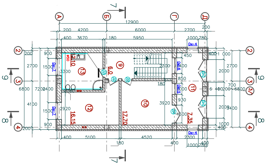
План 2—20 этаж на отм. +3,400
