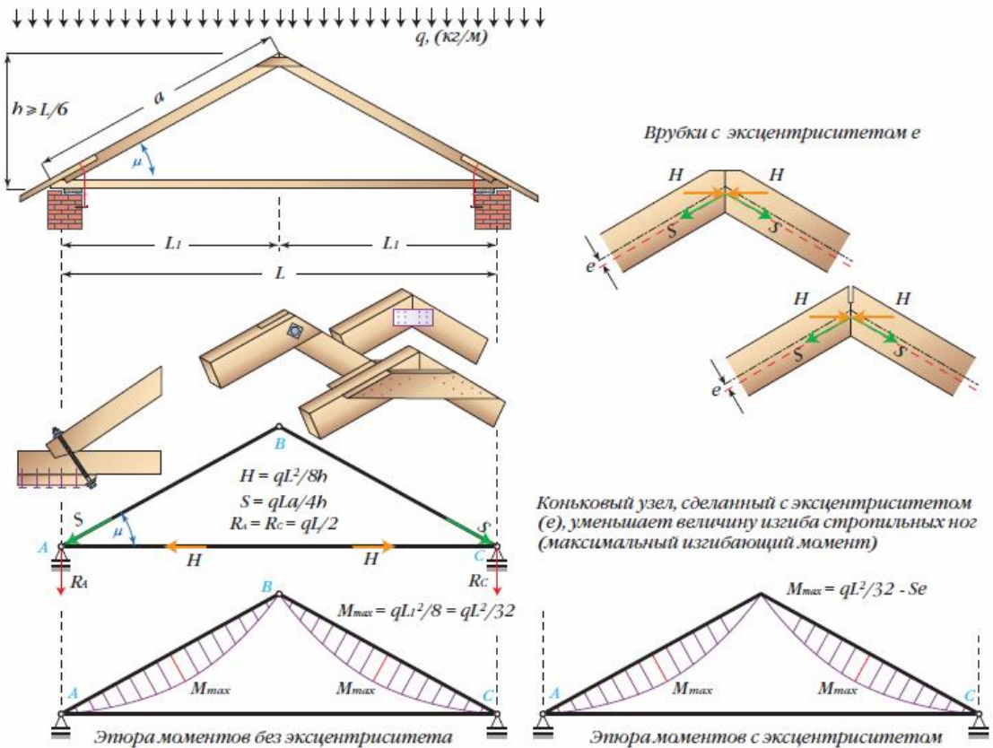
рис. 63. Трехшарнирная треугольная арка, расчетная схема висячих стропил
