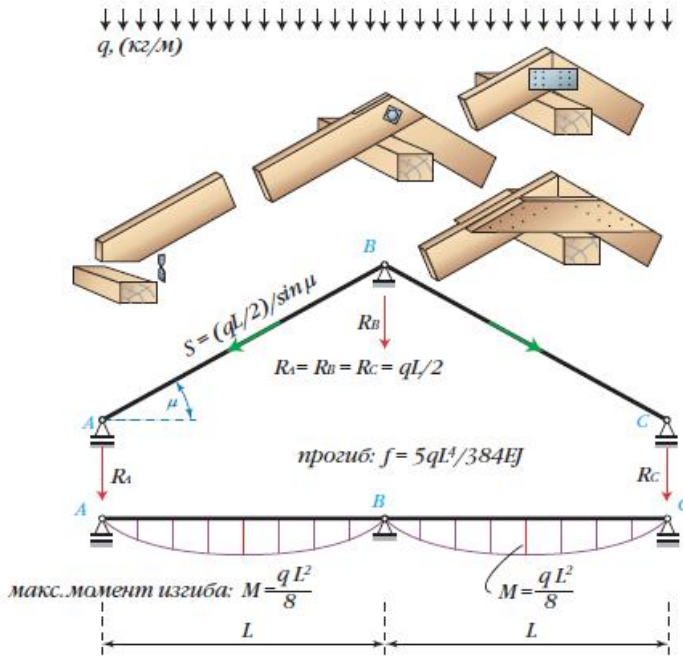
Рис. 33 Опираение низа стропил без врубки в мауэрлат с закреплением верха стропил, не дает распора на стены
