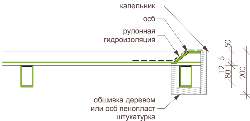
схема разреза
