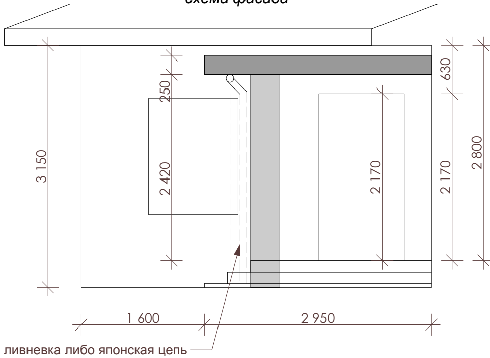
схема конструкций
