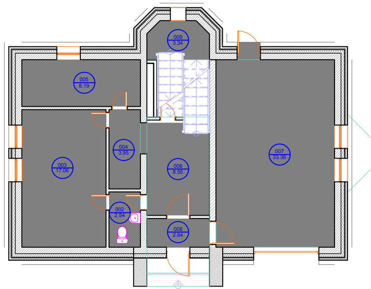
1. 1.Первый этаж 1:100
