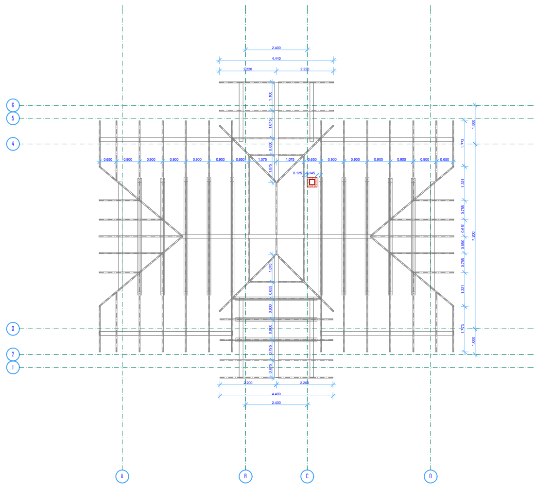
3. 3. Мансарда 1:100
