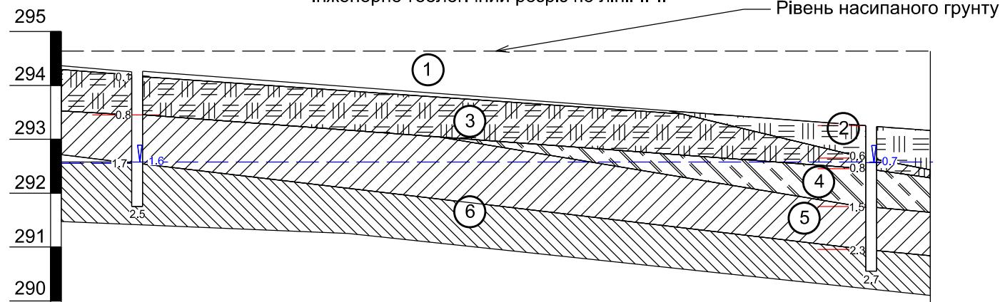
Інженерно-геологічний розріз по лінії II-II
