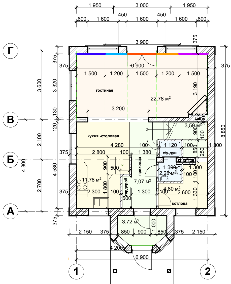
План на відмітці ±0,000. М 1:100
