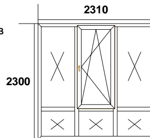
Позиция № 6 - ОКНО
