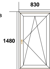
Позиция № 8 - ОКНО
