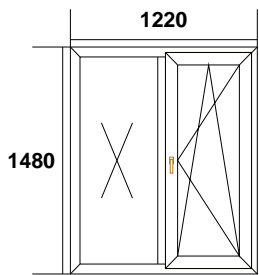
Позиция № 9 - ОКНО
