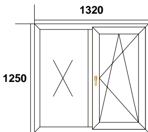
Позиция № 3 - ОКНО
