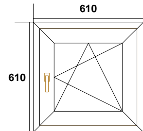
Позиция № 7 - ОКНО
