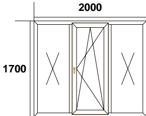
Позиция № 1 - ОКНО
