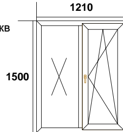
Позиция № 2 - ОКНО
