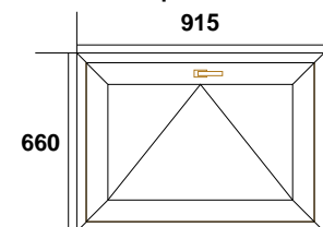
Позиция № 15 - ОКНО
