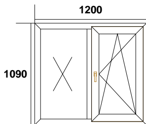
Позиция № 11 - ОКНО
