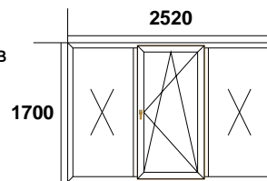
Позиция № 12 - ОКНО
