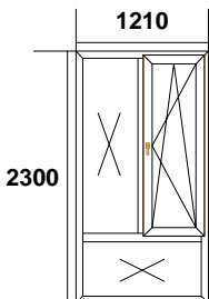
Позиция № 5 - ОКНО
