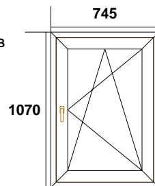
Позиция № 4 - ОКНО
