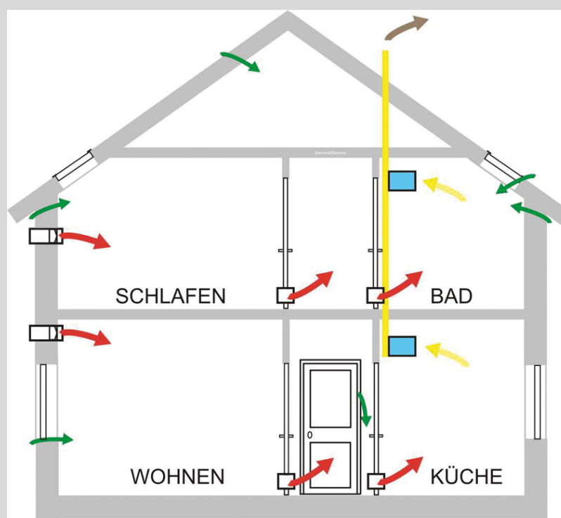
Abb. 5.6: Dezentrales Abluftsystem. Quelle: HEA
