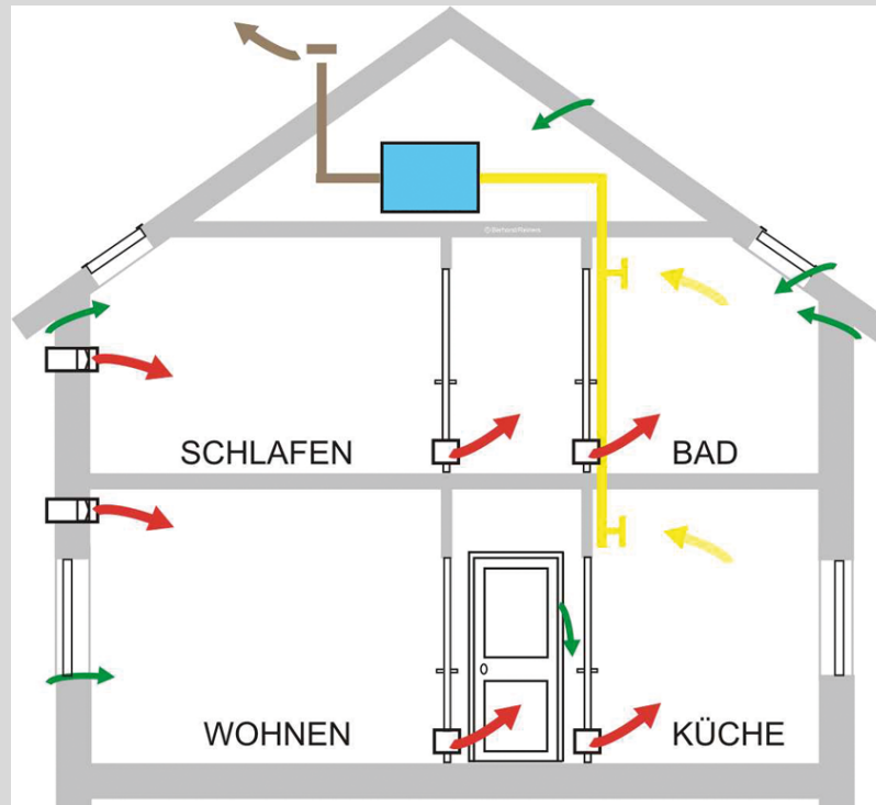
Abb. 5.5: Zentrales Abluftsystem. Quelle: HEA
