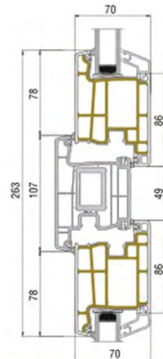
КОМБИНАЦИЯ ОКОННАЯ СТВОРКА И ДВЕРНАЯ СТВОРКА
