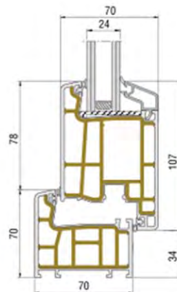
КОМБИНАЦИЯ РАМА ДВЕРНАЯ И СТВОРКА
