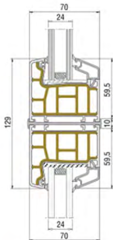
КОМБИНАЦИЯ РАМА И СОЕДИНИТЕЛЬНЫЕ ПРОФИЛИ
