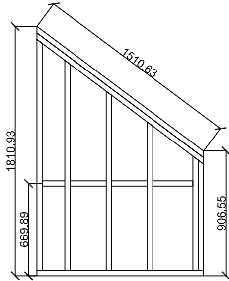
Détails murs
