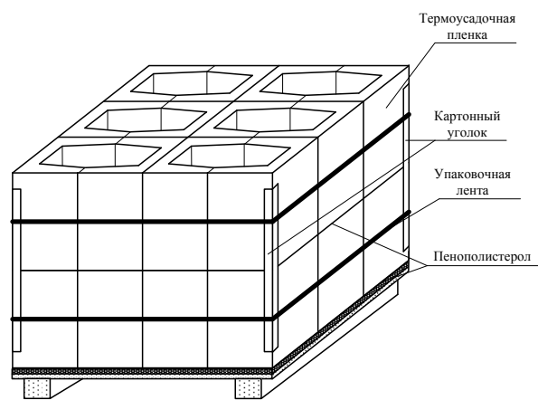
Вид собранного поддона U-блоков 200, 250
