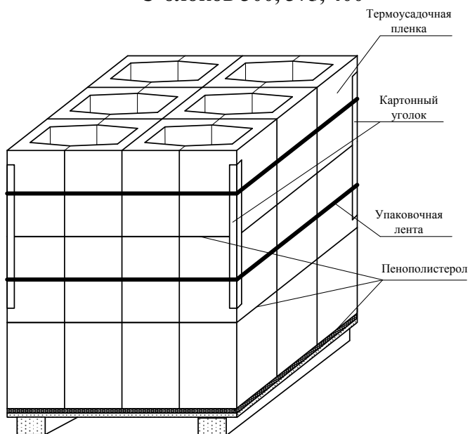
Вид собранного поддона U-блоков 300, 375, 400
