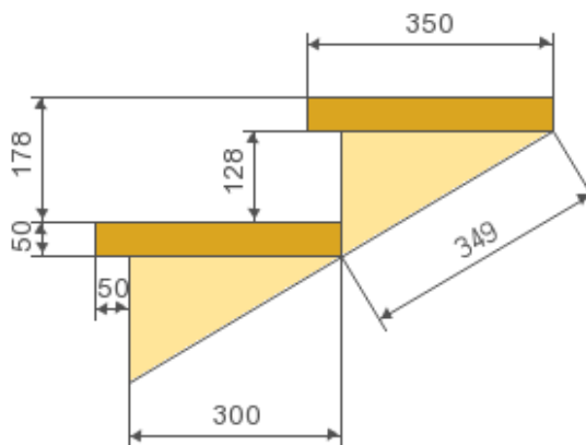
Чертеж шаблона ступеней
