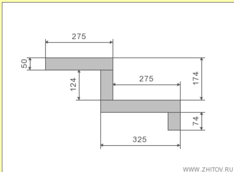
Розміри деталей тятиви
