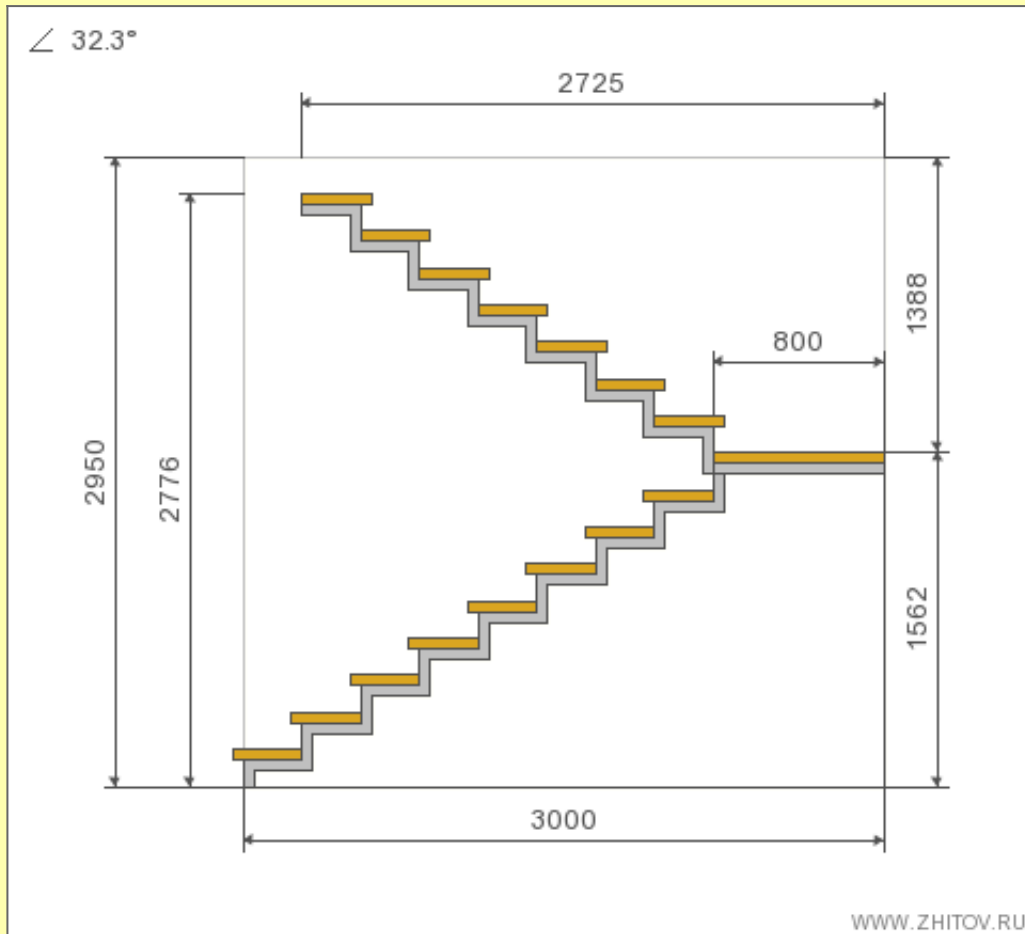
Загальне креслення сходів
