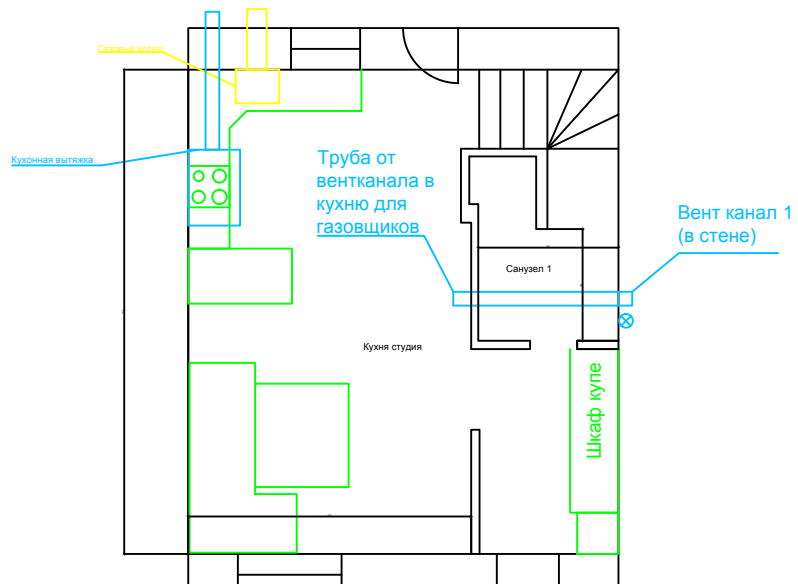
План 1-го этажа
