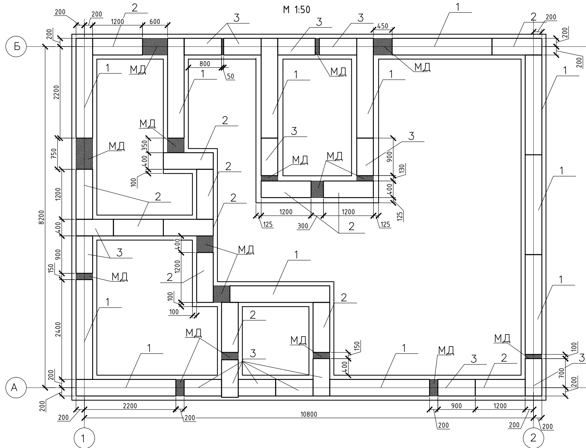
Специфікація на блоки ФБС другого ряду
