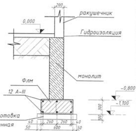
Сечение фундаментов 2-2
