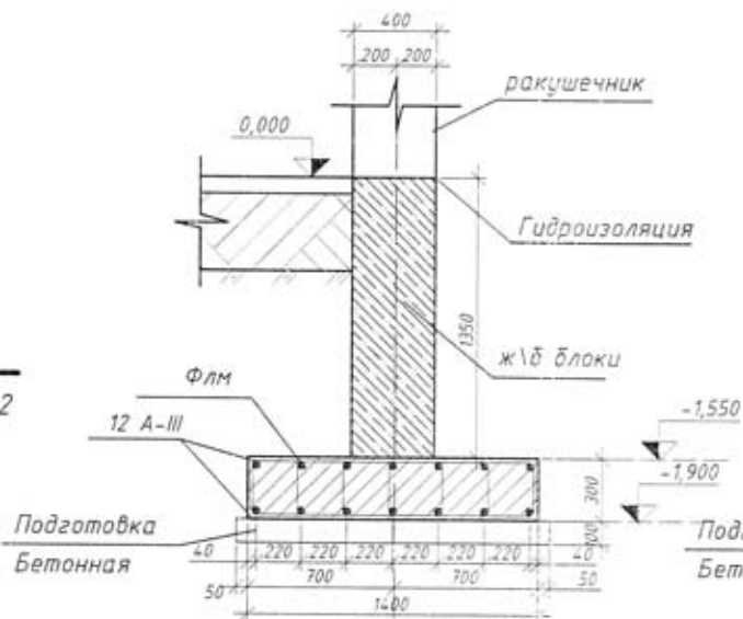
Сечение фундаментов 1-1
