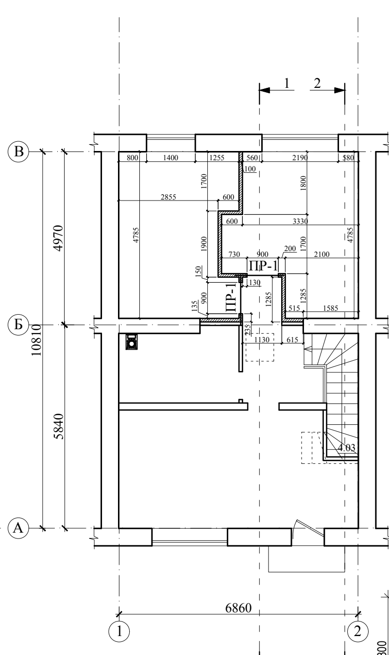
План 2-го поверху
