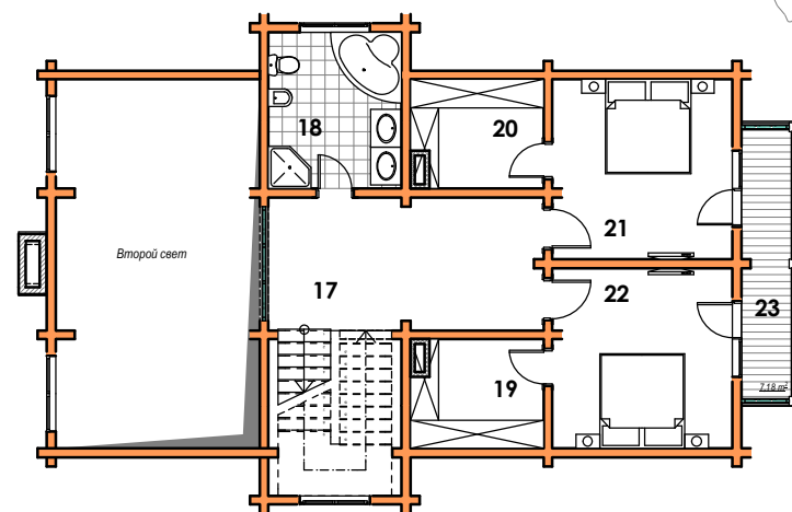
План на отм. +3.100
