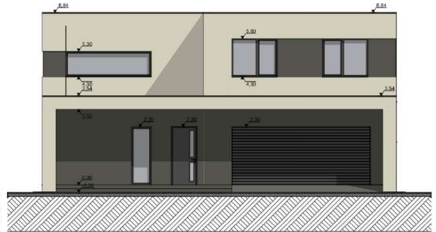
Фасад 1-2
