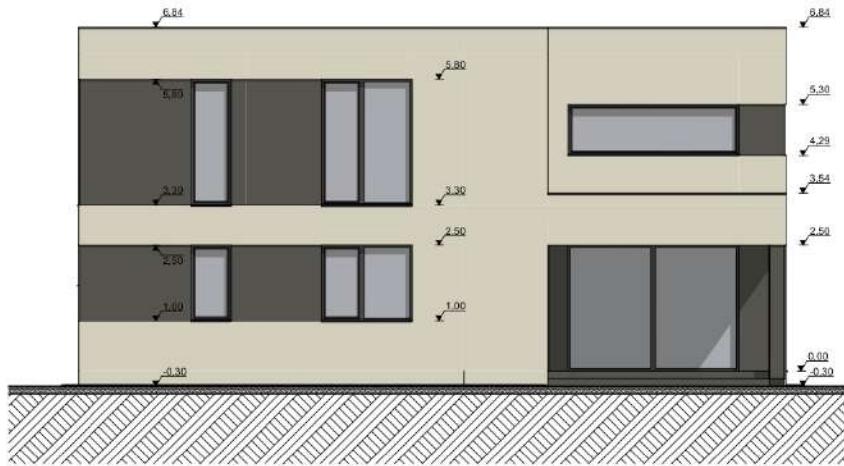
Фасад 3-3
