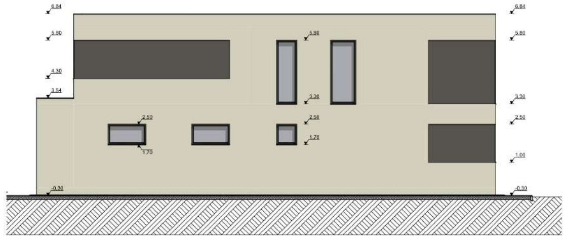
Фасад 4-4
