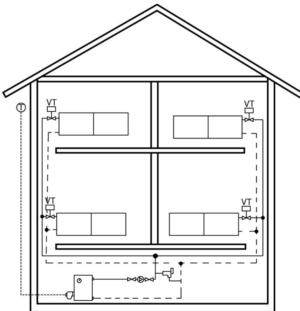
Рисунок 10 Пример 5 (По сравнению со схемой на рис.6 произведена комплексная модернизация системы отопления)
