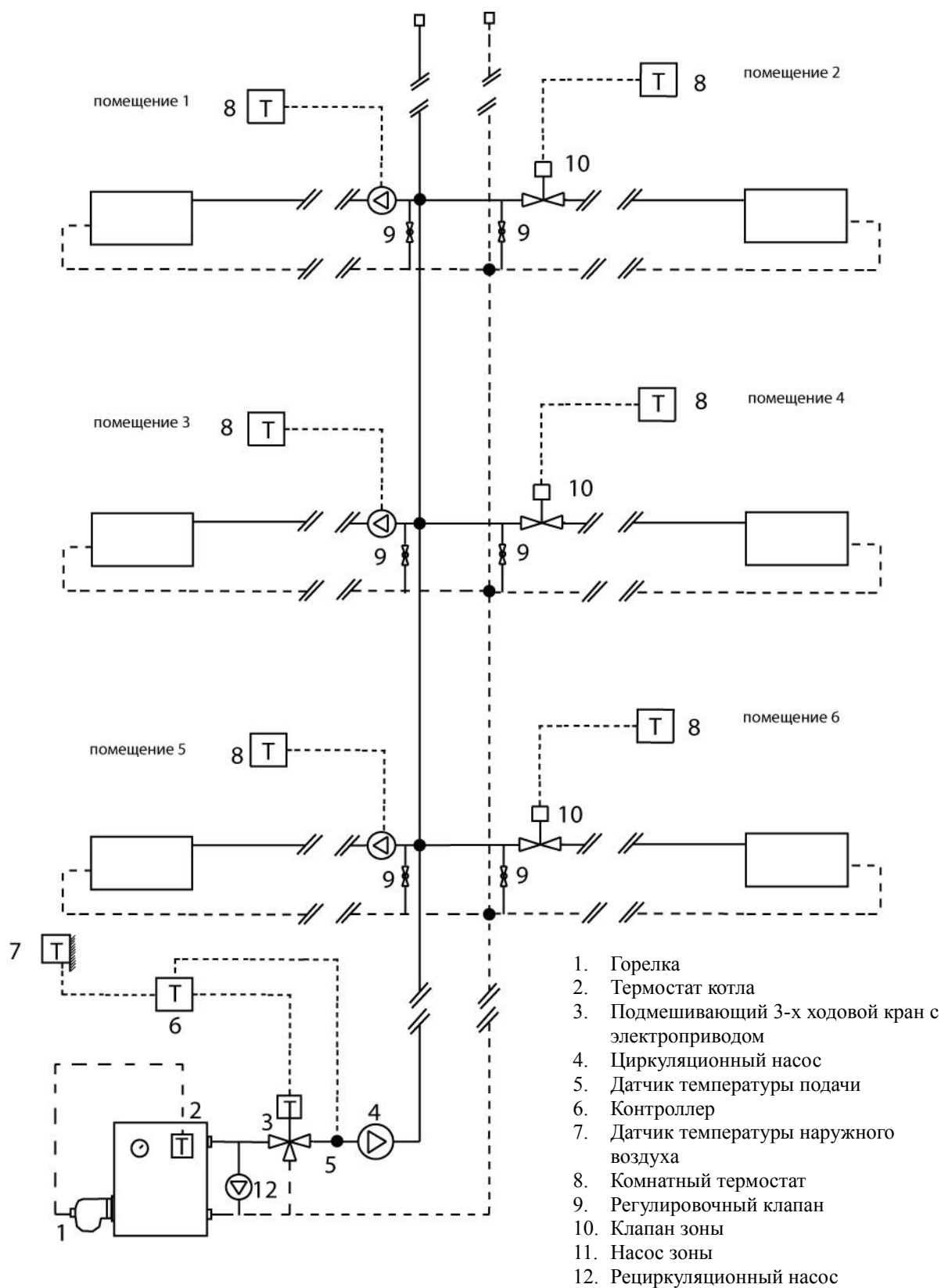
Рисунок 3 Схема типичной схемы отопления (70 годы)
