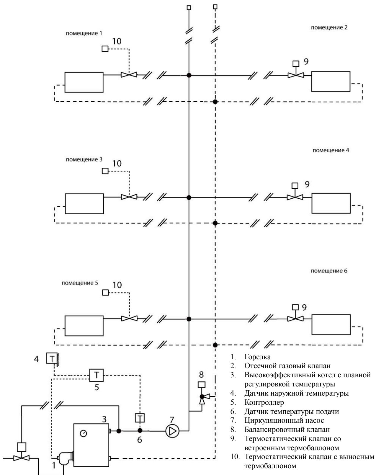
Рисунок 4 Схема типичной схемы отопления (современная)
