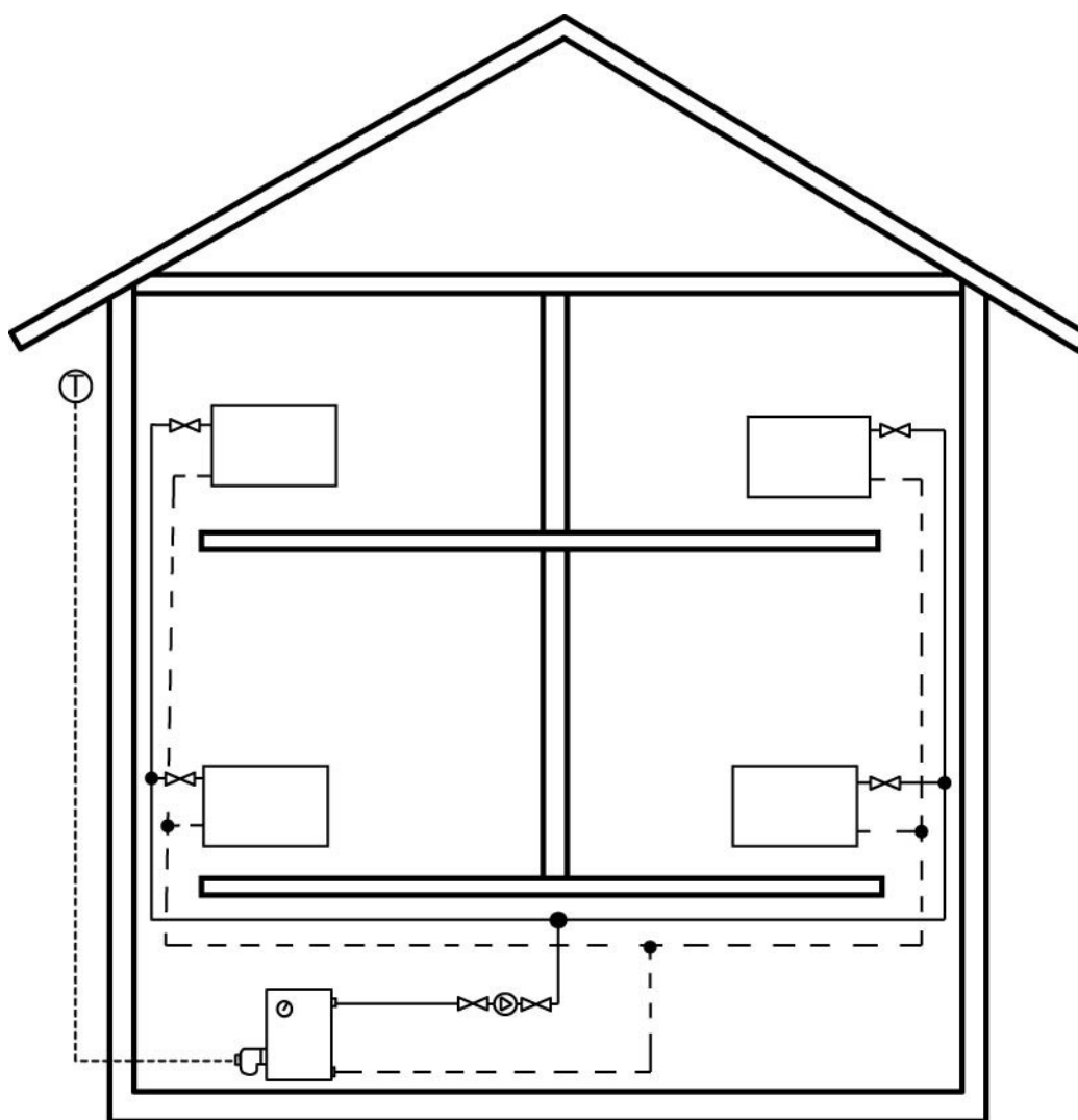
Рисунок 9 Пример 4 (По сравнению со схемой на рис.6 усовершенствовано производство тепла)
