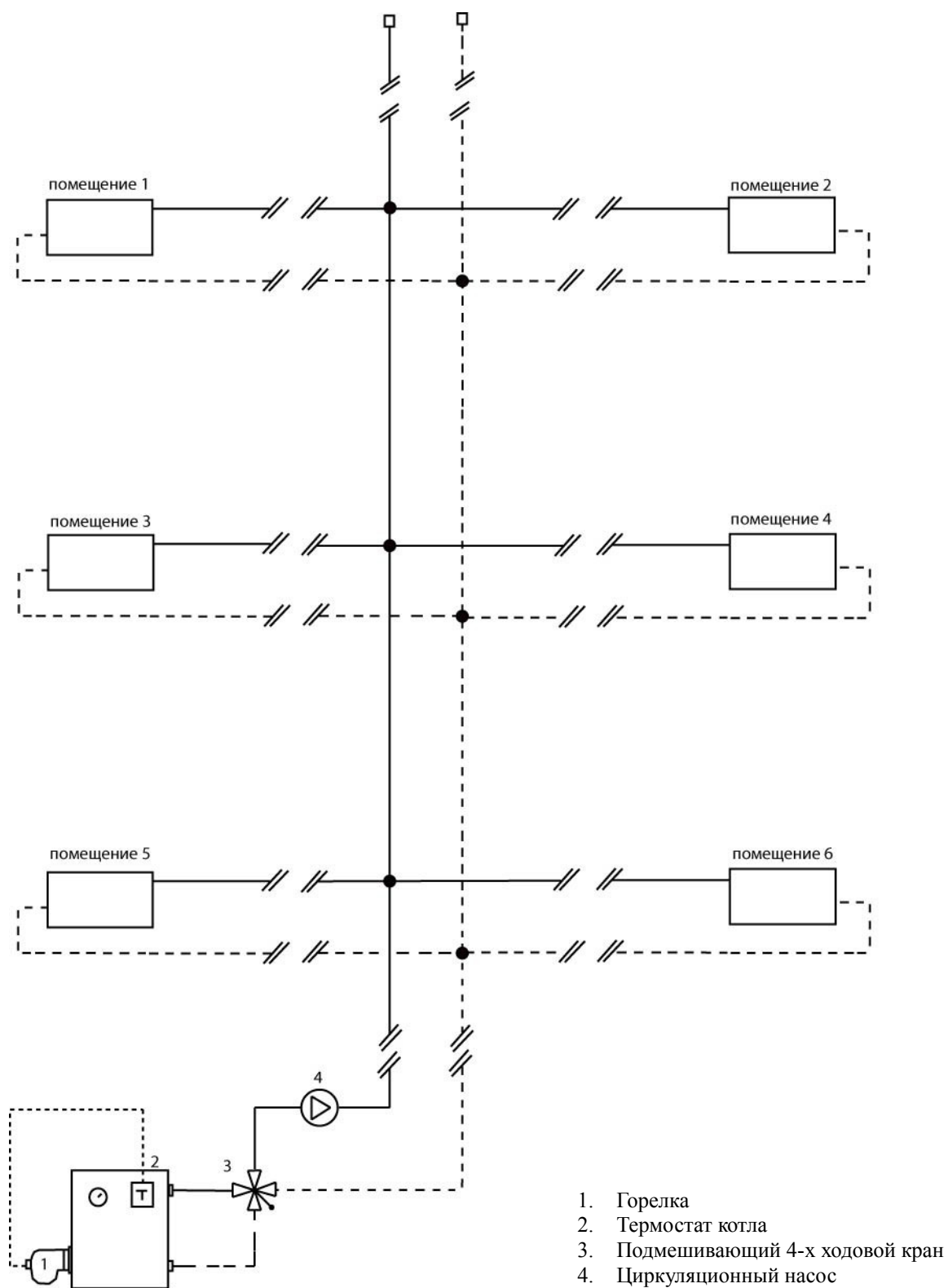
Рисунок 2 Схема типичной схемы отопления (60 годы)
