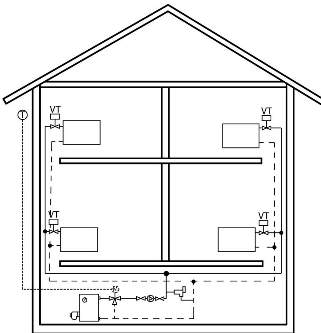
Рисунок 7 Пример 2 (По сравнению со схемой на рис.6 усовершенствовано регулирование системы)
