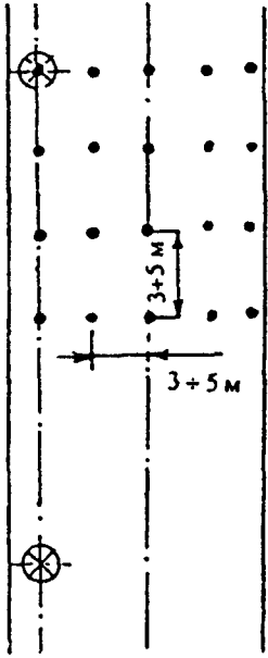
• — контрольная точка; ⊗ — светильник; Рисунок А4 — Расположение контрольных точек при измерении средней освещенности улиц при одностороннем однорядном расположении светильников
