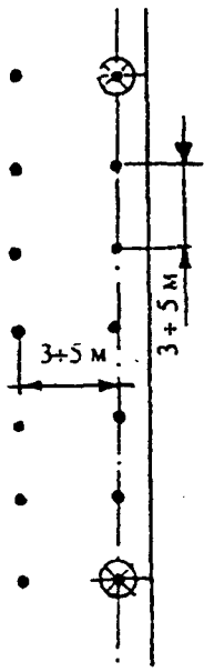
• — контрольная точка; ⊗ — светильник; Рисунок А5 — Расположение контрольных точек при измерении средней освещенности улиц при двух-стороннем прямоугольном расположении светильников
