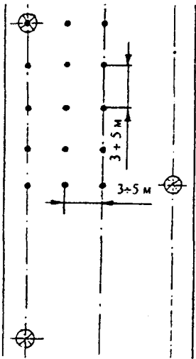
• — контрольная точка; ⊗ — светильник; Рисунок А6 — Расположение контрольных точек при измерении средней освещенности улиц при двухстороннем шахматном расположении
