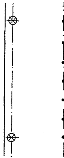
• — контрольная точка; ⊗ — светильник; Рисунок А7 — Расположение контрольных точек при измерении средней освещенности улиц при осевом однорядном расположении светильников
