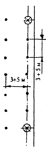
• — контрольная точка; ⊗ — светильник; Рисунок А7 — Расположение контрольных точек при измерении средней освещенности улиц при осевом однорядном расположении светильников
