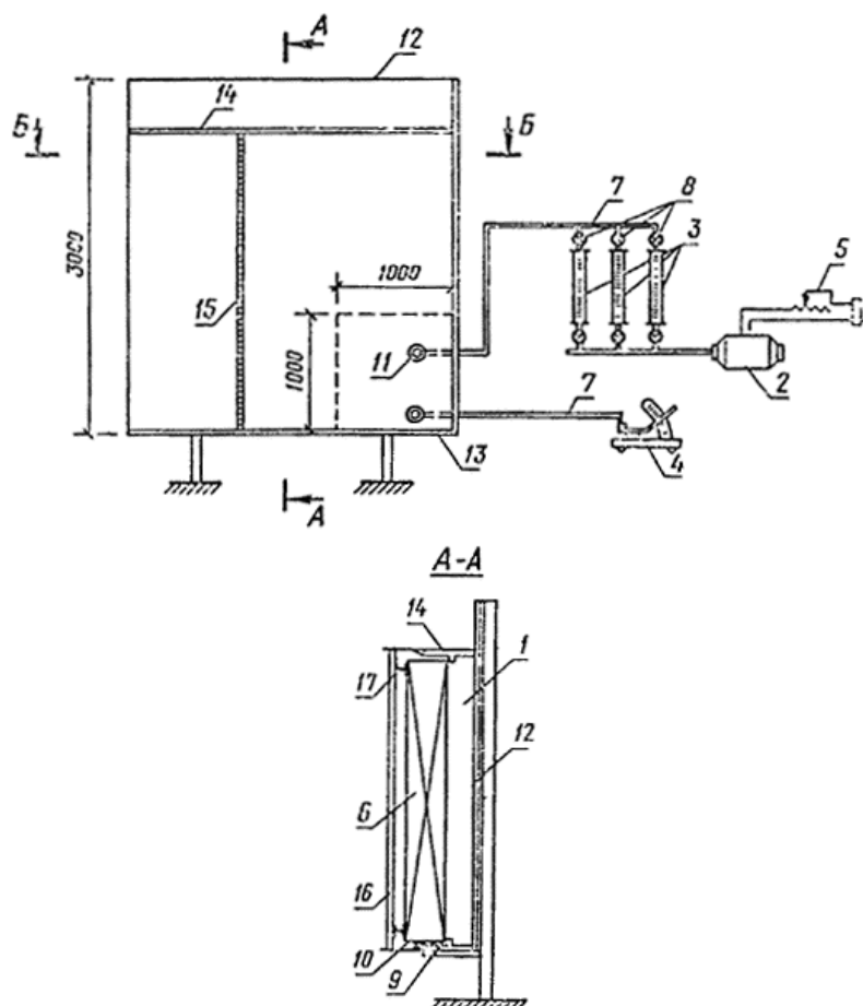
Схема установки для определения сопротивления воздухопроницанию ограждающих конструкций в лабораторных условиях
