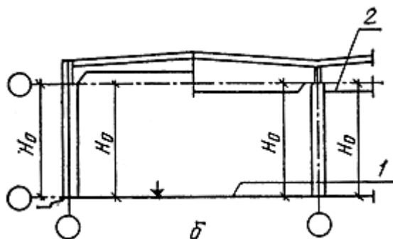
1 - координационная плоскость чистого пола; 2 - подвесной потолок
