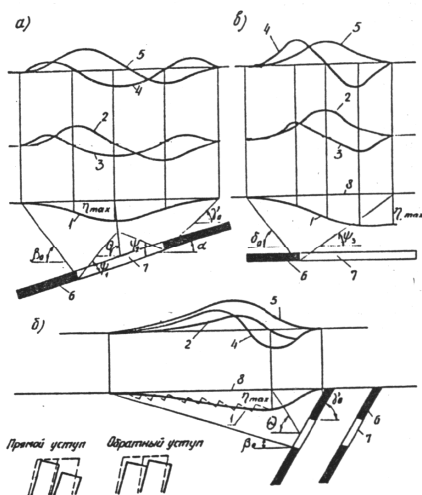
Черт. 1. Виды сдвигений и деформаций земной поверхности
