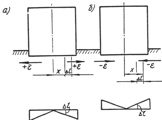
Черт. 2. Схемы к расчету перемещению точек земной поверхности под воздействием горизонтальных деформаций а — растяжению; б — сжатию
